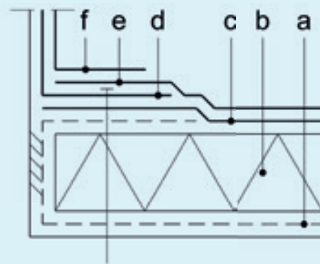
Voorbeeld detail uit Vakrichtlijn: PE laag bij bitumen dakbedekkingssystemen
